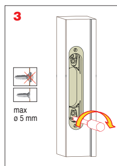
Монтаж регулируемой базы в дверную коробку; ВАЖНО: Самонарезающийся винт потайная плоская головка
