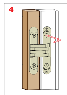
Монтаж петли в дверную коробку
