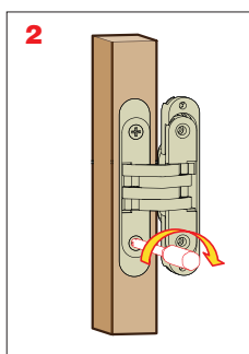
Монтаж фиксированной базы и петли в двери
