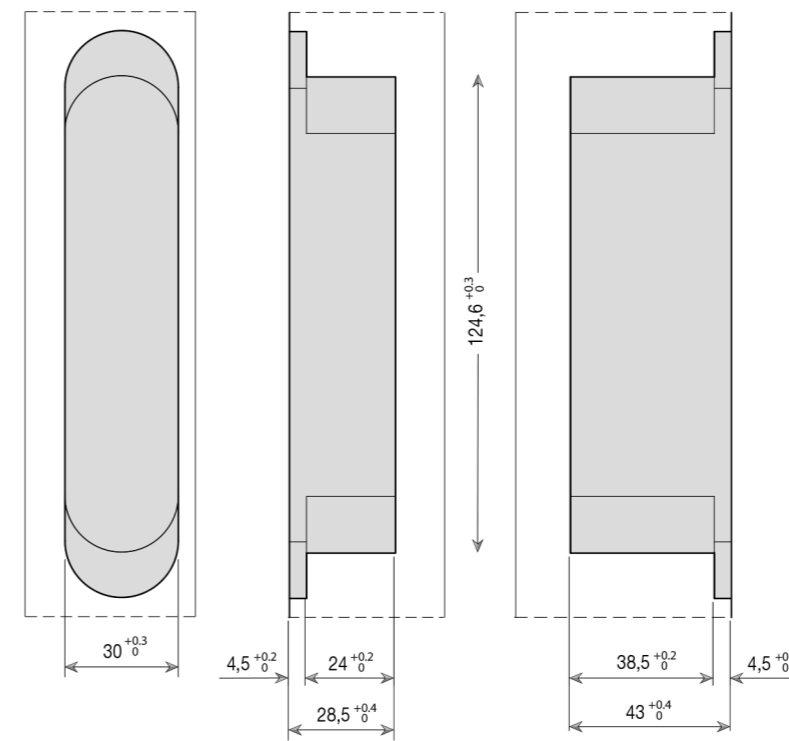
Чертеж в разрезе двери без четверти
